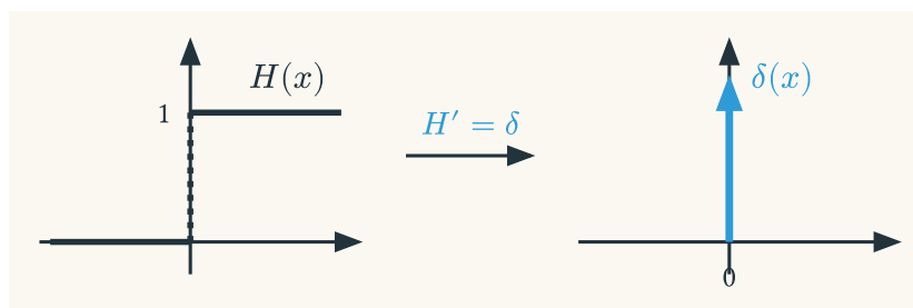
Рис. 1. Ступенька Хевисайда скачком переходит с 0 на 1; её обобщённая производная — дельта-импульс Дирака: бесконечно узкий и высокий пик ровно в точке скачка.
