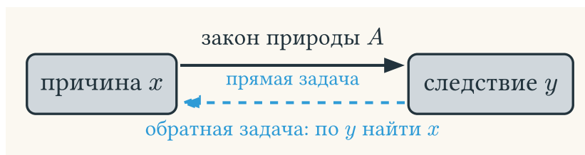
Рис. 1. Прямая задача идёт по стрелке закона природы: причина \rightarrow следствие. Обратная задача идёт против стрелки — по наблюдаемому последствию восстановить скрытую причину.
