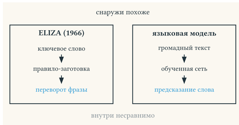
Рис. 1. Слева ELIZA: ключевое слово запускает правило-заготовку, и фраза переворачивается обратно вопросом. Справа языковая модель: ответ рождается как предсказание следующего слова обученной сетью. Снаружи похоже, внутри несравнимо.
